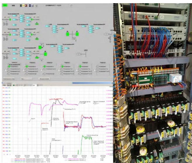
ПТК Minigrd разработан, спроектирован, изготовлен, протестирован и смонтирован на электродинамической модели НИУ МЭИ
